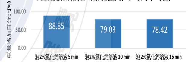
海藻酸鈉紙吸管的耐濕性質(2小時內平均值)
