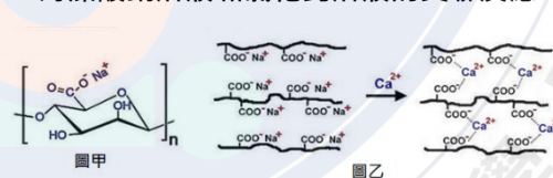
海藻酸鈉溶液和氯化鈣溶液的交聯反應
