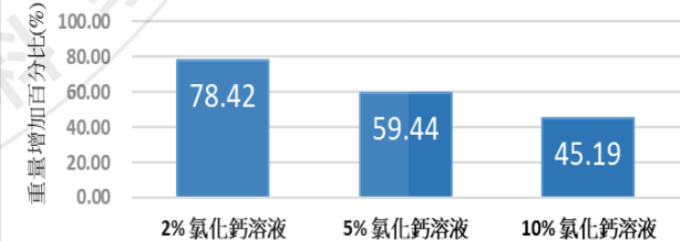
海藻酸鈉紙吸管的耐濕性質測試(2小時內平均值)
