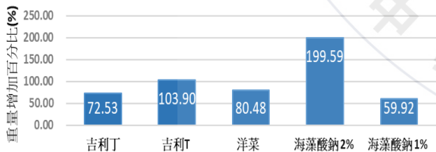
紙吸管的耐濕性質測試(2小時內平均值)
