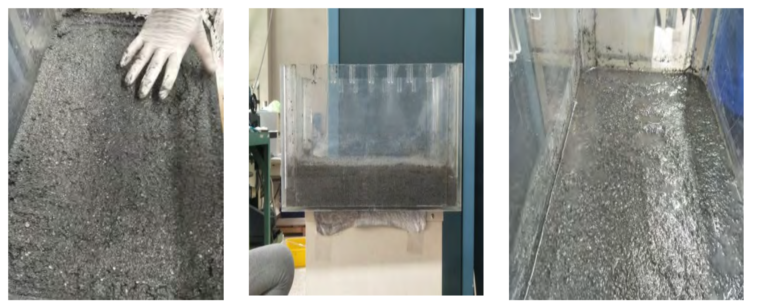
圖十四、實驗準備3000ml水以砂土加入直到表層無水光反射視為飽和砂土
