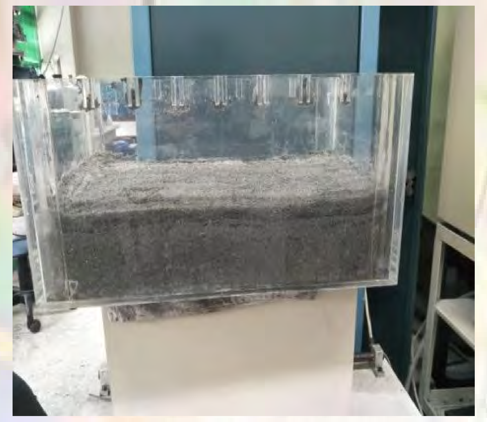
圖十二 土壤液化實驗器材 透明壓克力箱、砂石及搖擺爐
