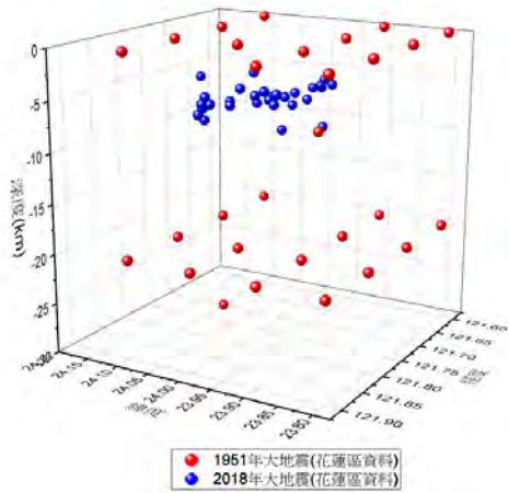
圖十八、1951 與 2018 花蓮大地震 規模四以上震源立體分佈
