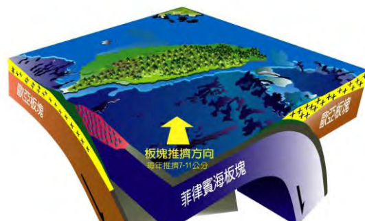
圖一 台灣板塊運動示意圖
