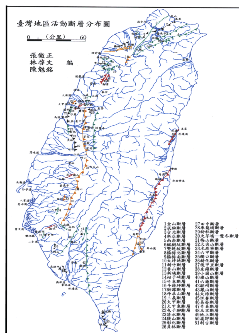
圖三 台灣地區活動斷層分佈圖
