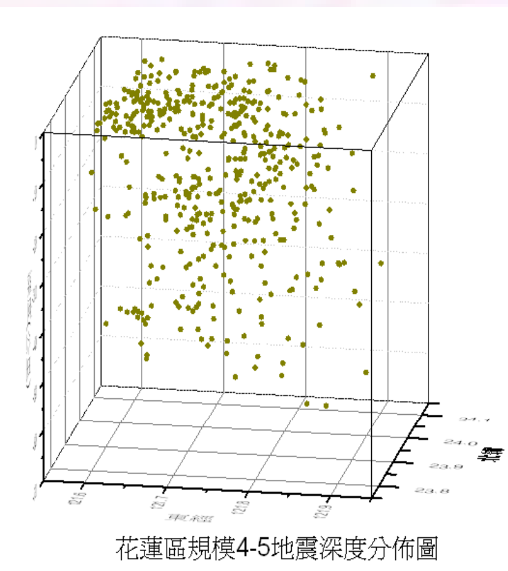
圖七 摘自震震七星潭 -花蓮縣科展作品
