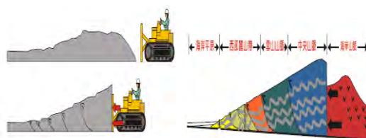
圖二 板塊推擠產生斷層示意圖
