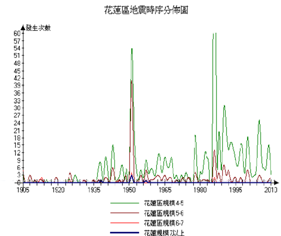
圖十 摘自震震七星潭 -花蓮縣科展作品
