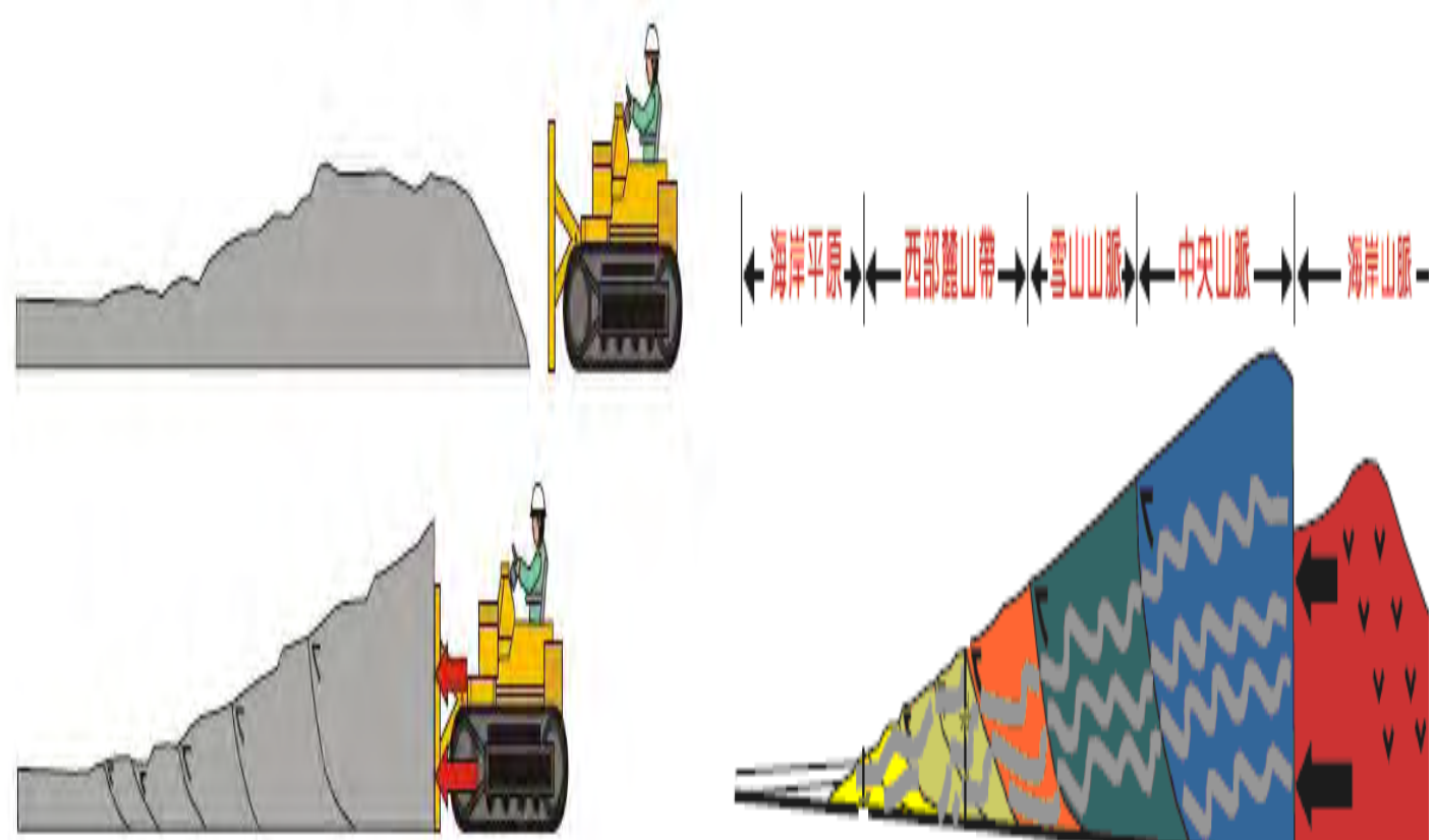
圖二 板塊推擠產生斷層示意圖 摘自國家地震工程研究中心認識地震工程手冊
