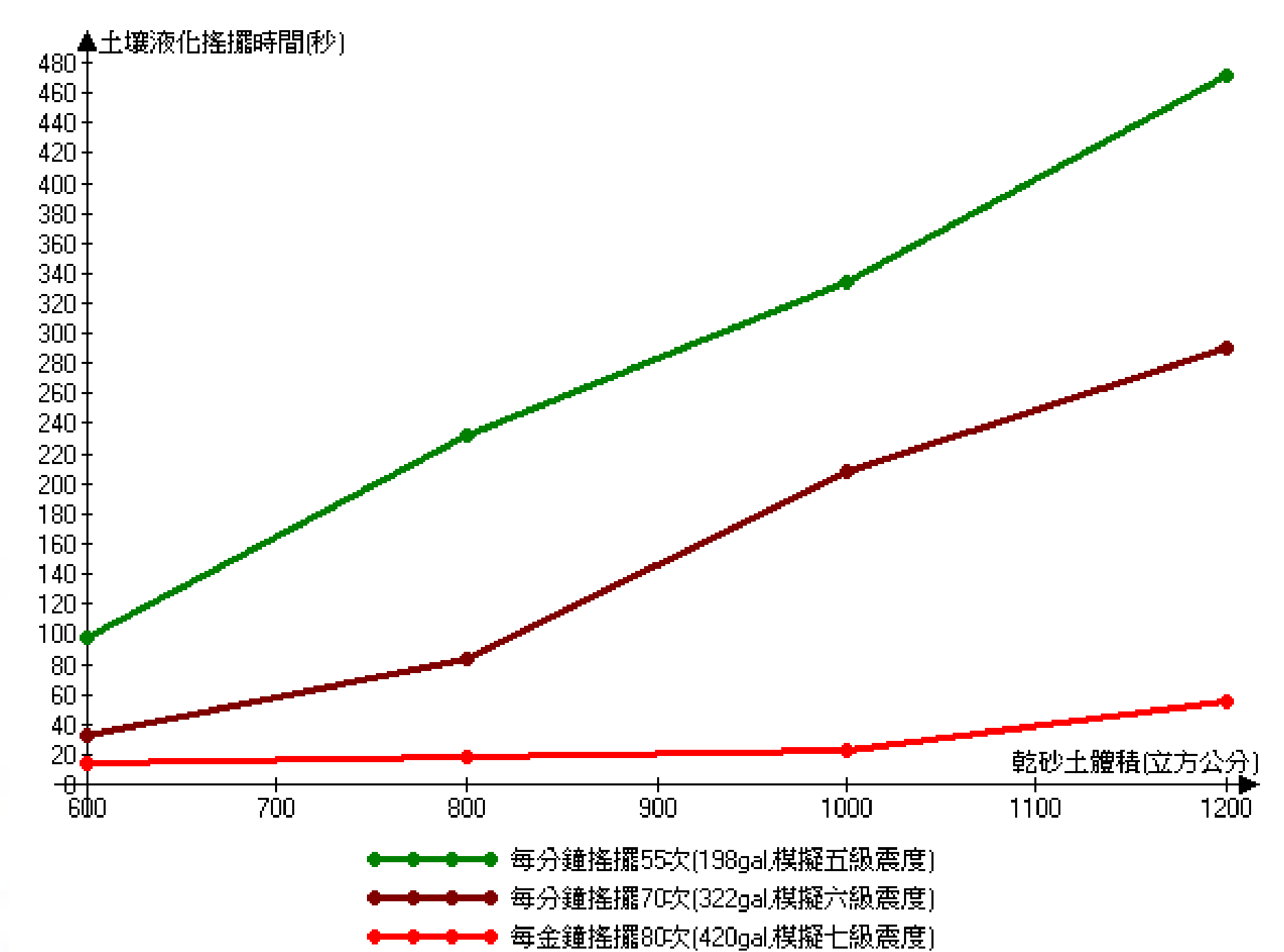
土壤液化實驗結果
