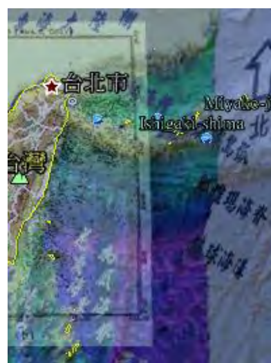
圖五 規模 4 以上地震分佈
