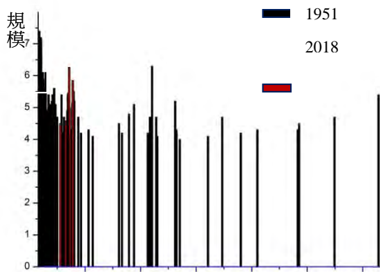
圖十九、1951 與 2018 花蓮大地震 規模四以上時序分佈圖
