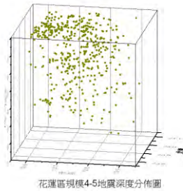
圖七 摘自震震七星潭 -花蓮縣科展作品(2011)
