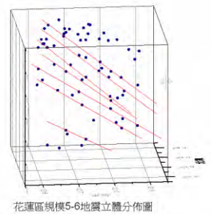
圖八 摘自震震七星潭 -花蓮縣科展作品(2011)
