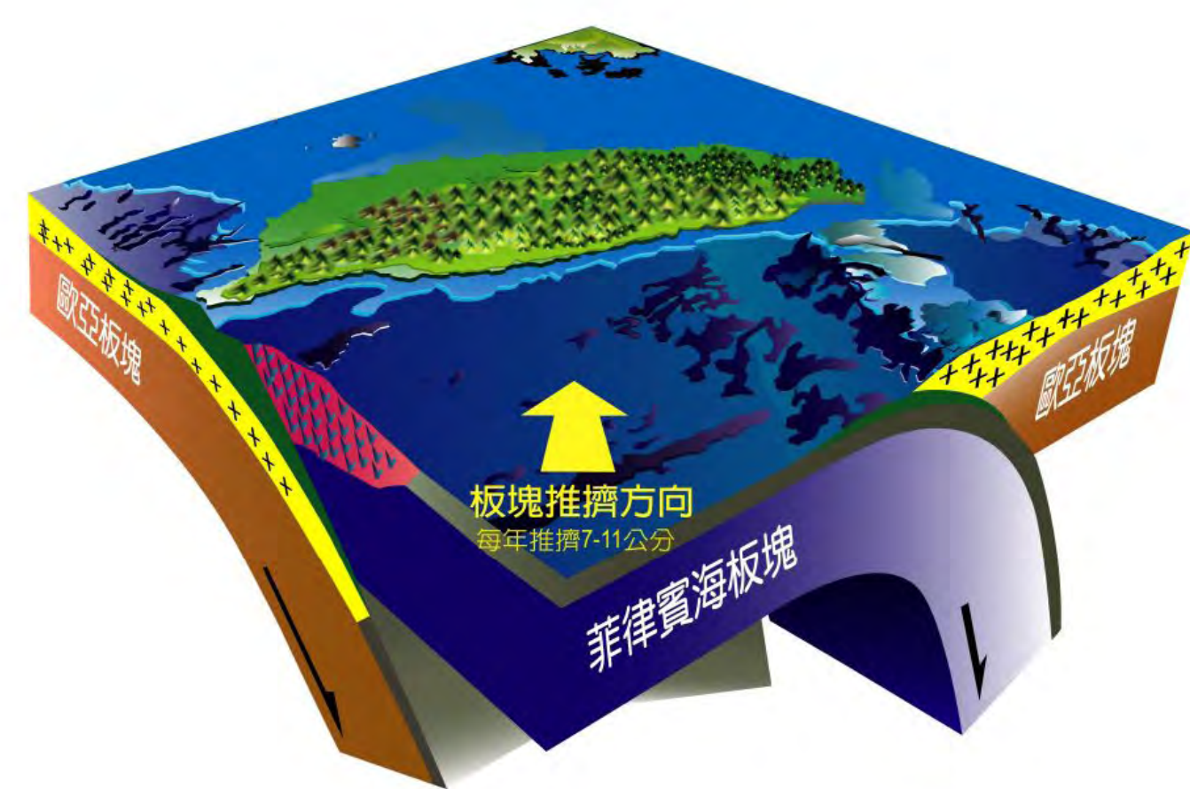
圖一 台灣板塊運動示意圖 摘自國家地震工程研究中心認識地震工程手冊
