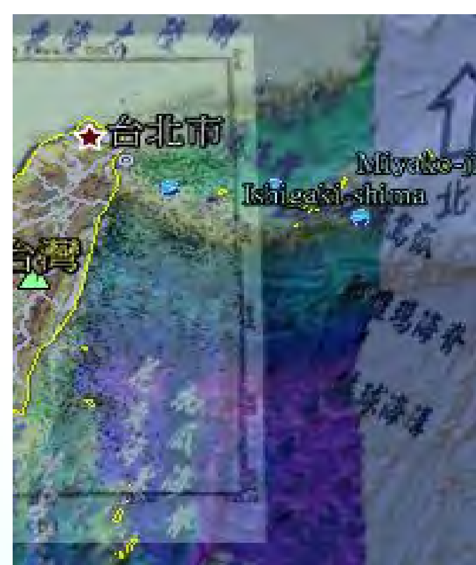
圖五 規模4以上地震分佈 (疊合海域數值地形圖)
