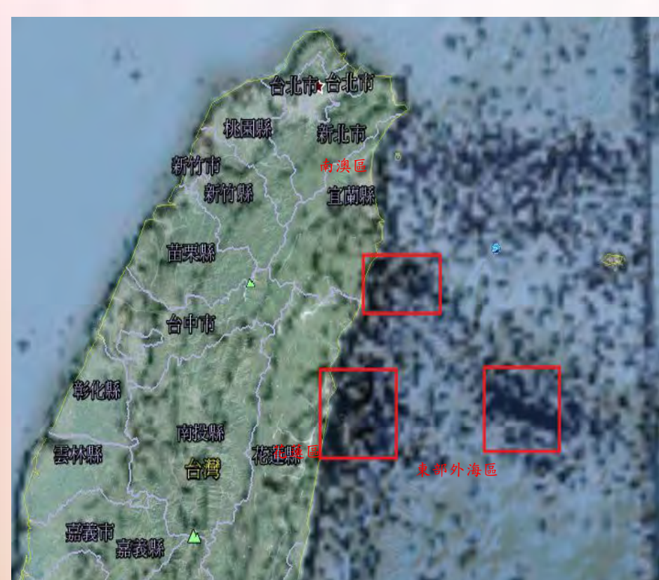
圖六 花蓮外海大三角 摘自震震七星潭 -花蓮縣科展作品
