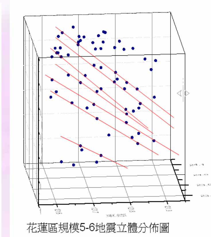
圖八 摘自震震七星潭 -花蓮縣科展作品
