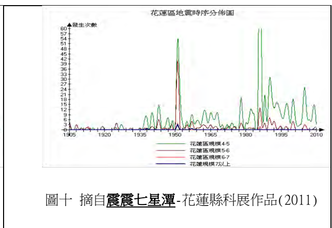
圖九 摘自震震七星潭-花蓮縣科展作品(2011)
