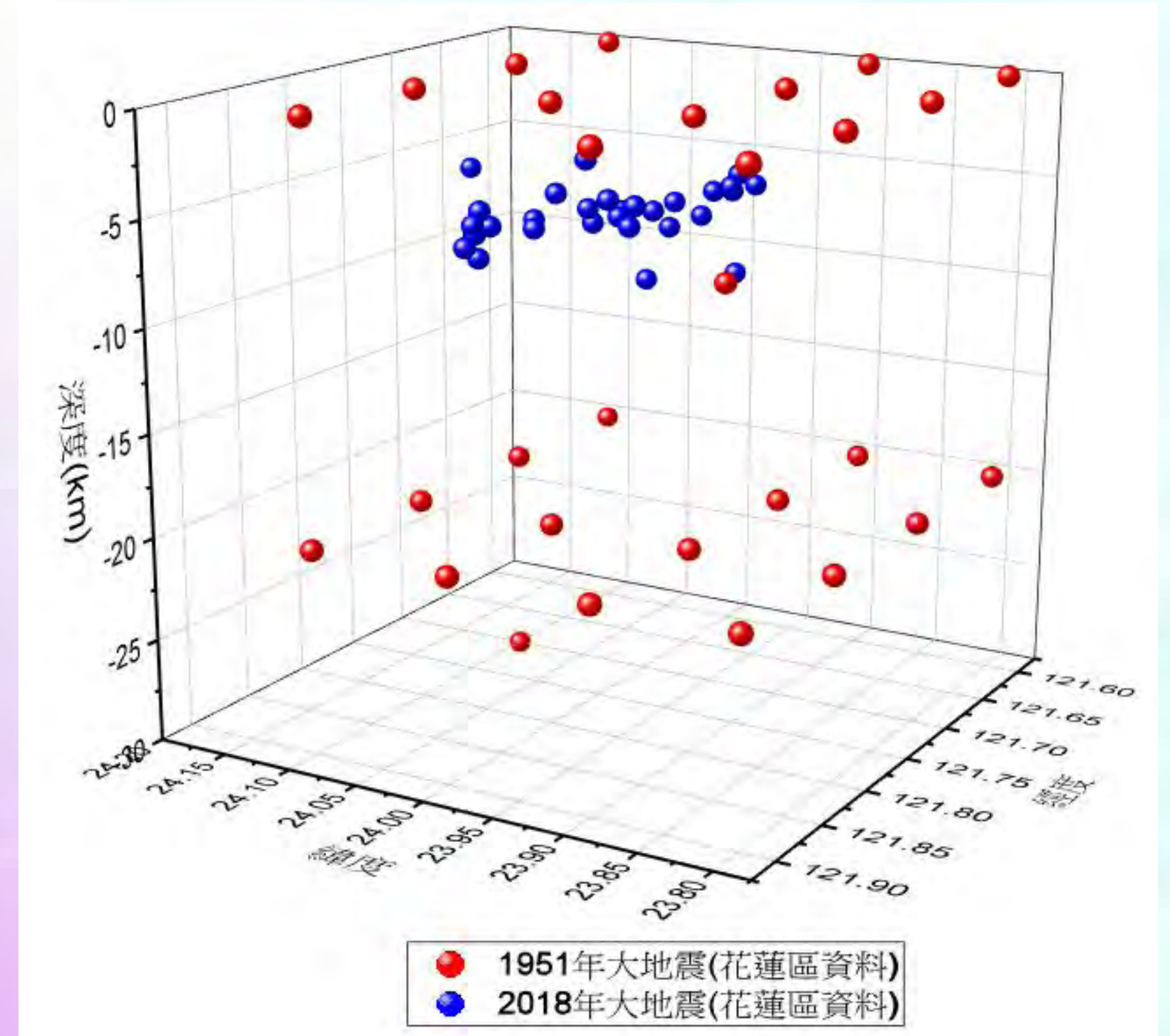
圖十八、1951與2018花蓮大地震規模四以上震源立體分布
