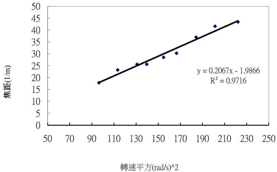
圖 9 轉速平方與焦距關係圖
